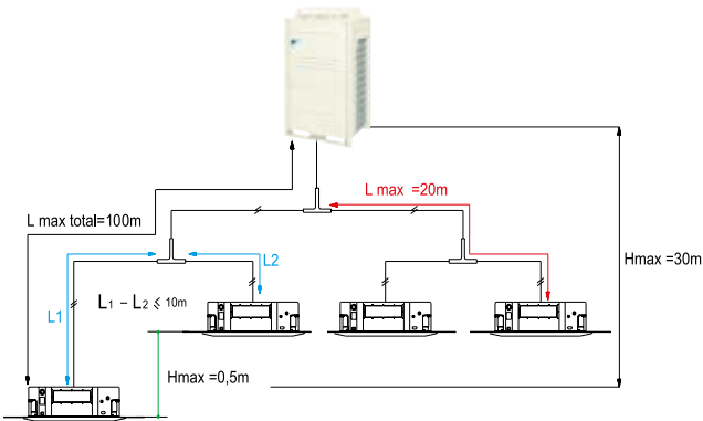
Esquema Doble Twin
