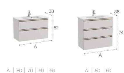
Lavabos compatibles con muebles base
