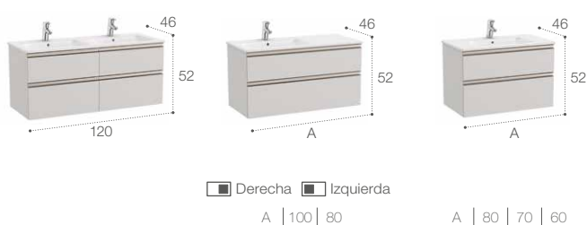
Unik compacto (lavabo y mueble)
