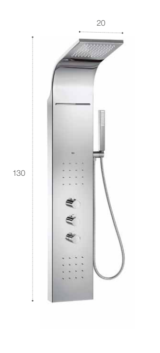
Columna de hidromasaje termostática exterior
