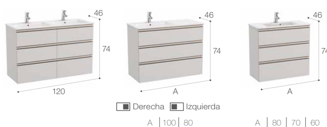
Mueble base para lavabo de sobre encimera
