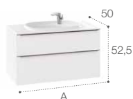
Unik (lavabo y mueble) con lavabo de Fineceramic® y apertura mediante tirador
