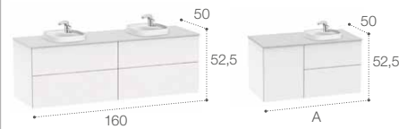
Mueble base para lavabo de encimera
