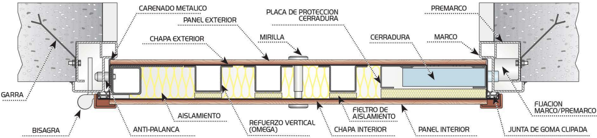
Sección horizontal
