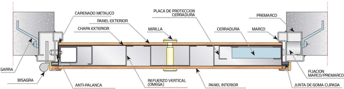
Sección horizontal
